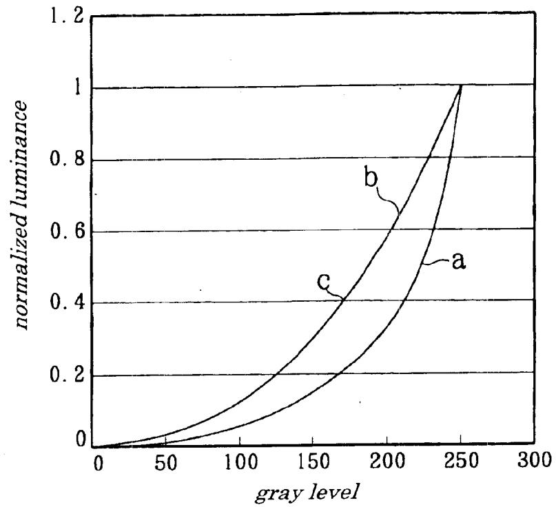
FIG.16(PRIOR ART)
