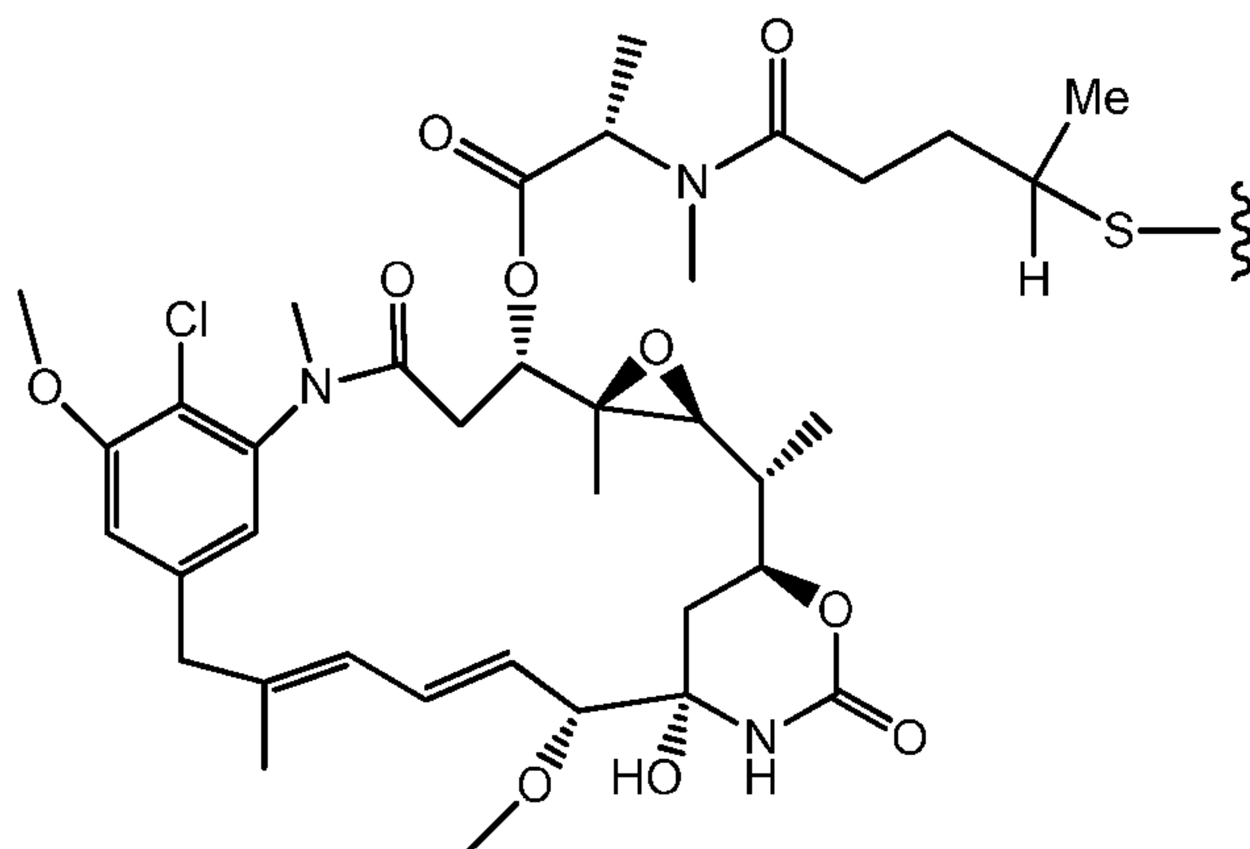
DM3
