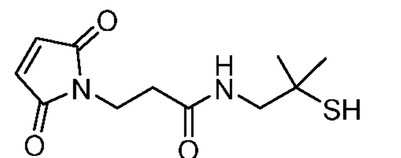
MPBT: maleimidoPropionamidoButylThio
