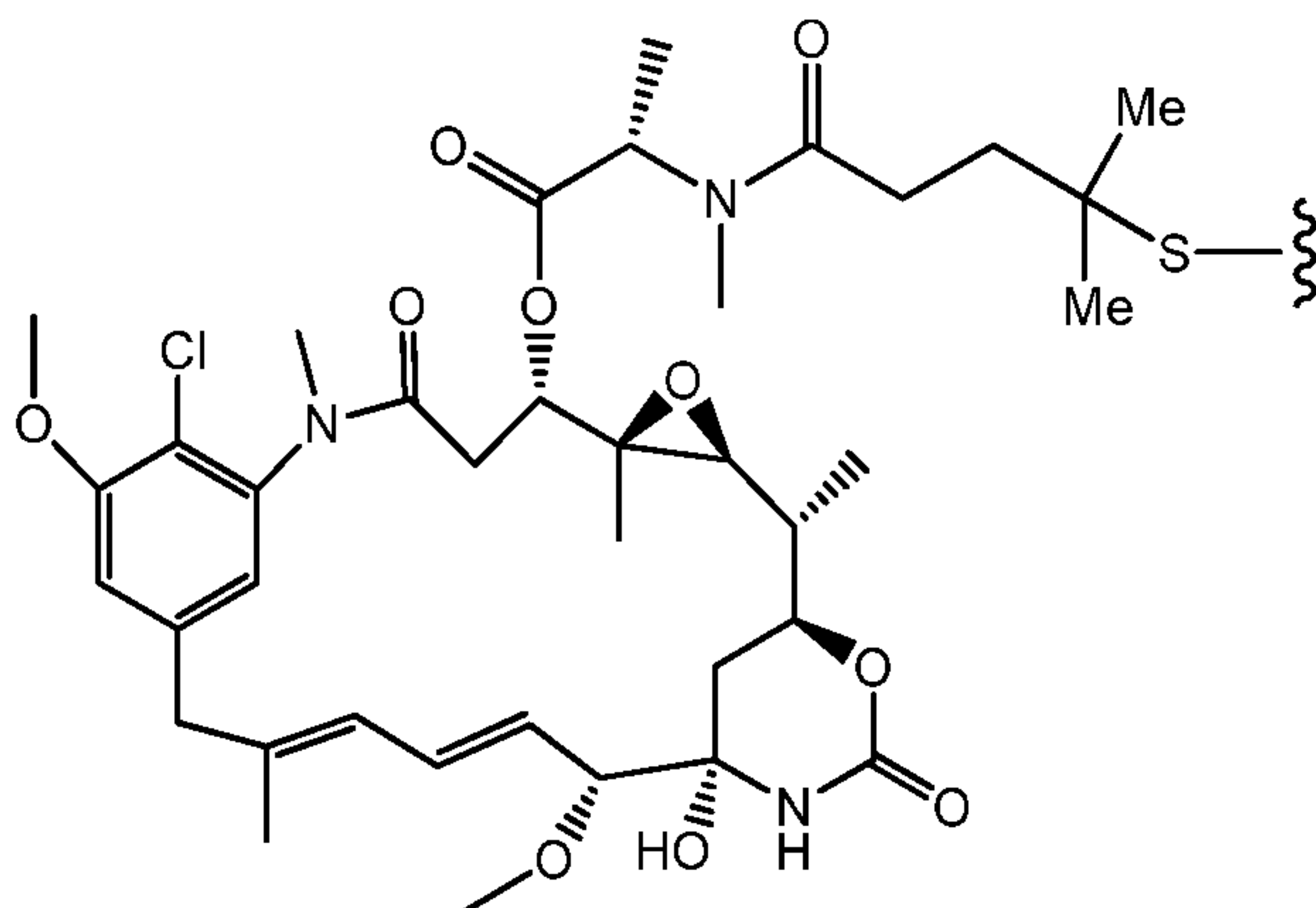
DM4
