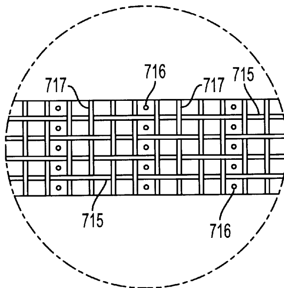
FIG. 8C
