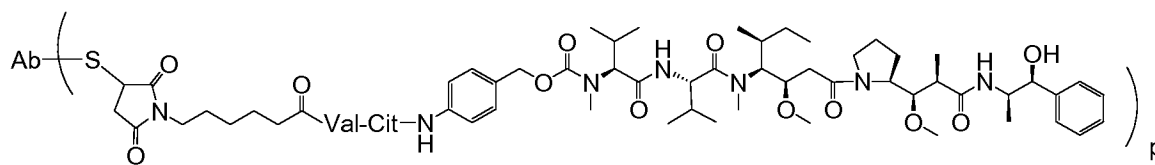
Ab-MC-vc-PAB-MMAE
