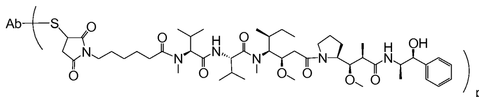
Ab-MC-MMAE
