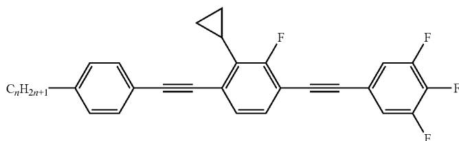
PTG(c3)TU-n-F
