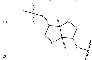
(dianhydroiditol)
