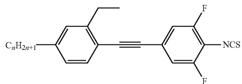
P(2)TU-n-S
