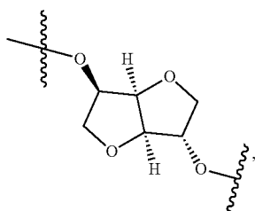
(dianhydrosorbitol)
