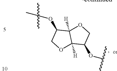
(dianhydromannitol)
