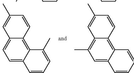
1,2-, 1,8-, 1,9-, 2,3-, 2,5- and 2,10-phenanthrylenes
