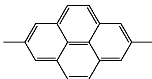
2,7-pyrenylene
