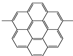
1,6-coronenylenes
