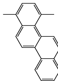
1,4-chrysenylene
