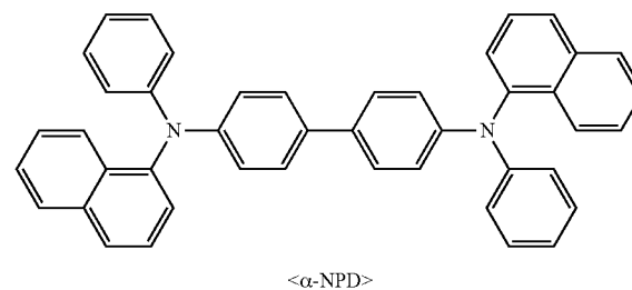
< \alpha -NPD>
