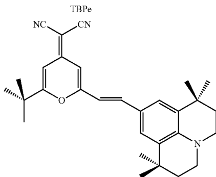
DCJTb
