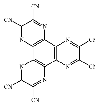
&lt;HAT-CN&gt;
