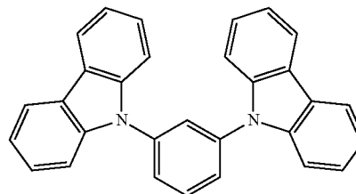
&lt;mCP&gt;
