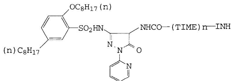
Compound No. 21B-No. 25B
