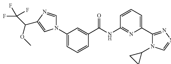
N-(6-(4-cyclopropyl-4H-1,2,4-triazol-3-yl)pyridin-2-yl)-3-(4-(2,2,2-trifluoro-1-methoxyethyl)-1H-imidazol-1-yl)benzamide
