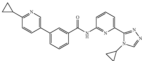
N-(6-(4-cyclopropyl-4H-1,2,4-triazol-3-yl)pyridin-2-yl)-3-(6-cyclopropylpyridin-3-yl)benzamide
