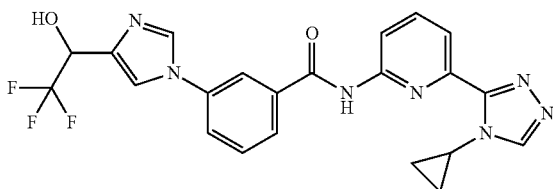
N-(6-(4-cyclopropyl-4H-1,2,4-triazol-3-yl)pyridin-2-yl)-3-(4-(2,2,2-trifluoro-1-hydroxyethyl)-1H-imidazol-1-yl)benzamide
