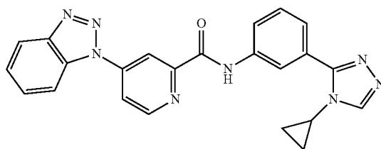
4-(1H-benzo[d][1,2,3]triazol-1-yl)-N-(3-(4-cyclopropyl-4H-1,2,4-triazol-3-yl)phenyl)picolinamide
