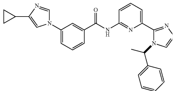
(R)-3-(4-cyclopropyl-1H-imidazol-1-yl)-N-(6-(4-(1-phenylethyl)-4H-1,2,4-triazol-3-yl)pyridin-2-yl)benzamide
