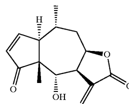
24. Ambrosin
