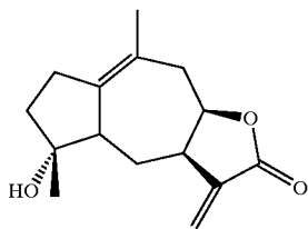
26. Pseudoivalin
