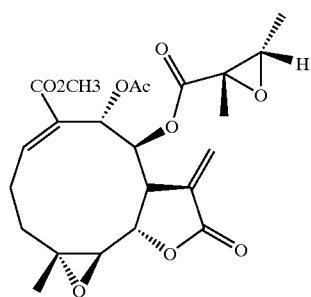
6. Enhydrin
