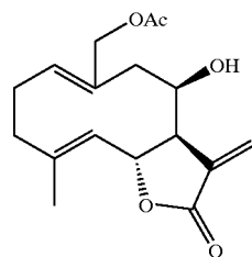
8. Ovatifolin
