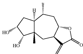
28. Gigerinin
