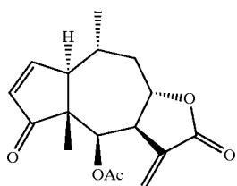
27. Linifolin A
