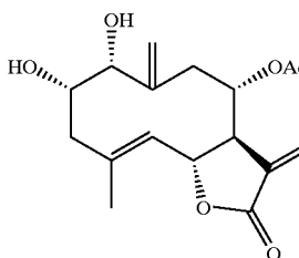
14. Verlotin
