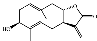
19. Chamissonin
