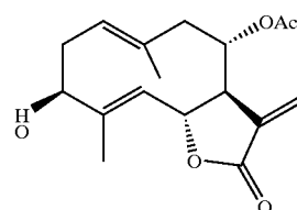
12. Chihuahuin
