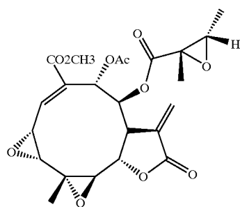
5. Leucanthin B
