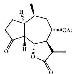
21. Confertiflorin
