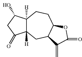
30. Burrodin
