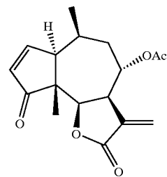
24. Ambrosin
