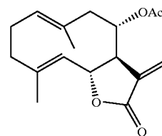
11. Tulipinolide
