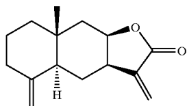
38. Isoalantolactone
