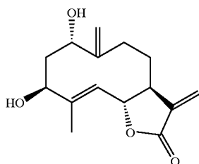
15. Artemarin
