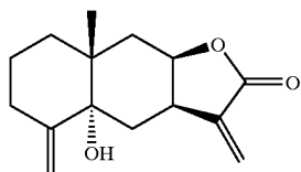
40. Telekin
