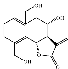
18. Albicolide
