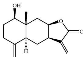
31. Asperilin
