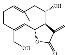
16. Salonenolide
