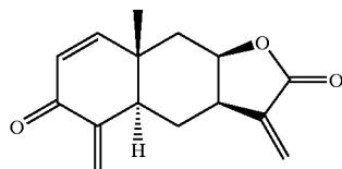
39. Encelin
