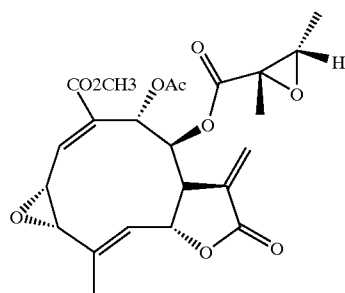
7. Melampodin A
