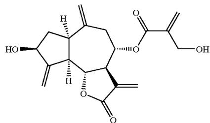
23. Cynaropicrin
