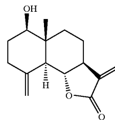
35. Reynosin
