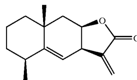
37. Alantolactone
