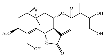
17. Eriophyllin
