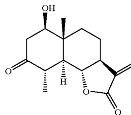
34. Artecadin
