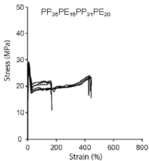
FIG. 22B
