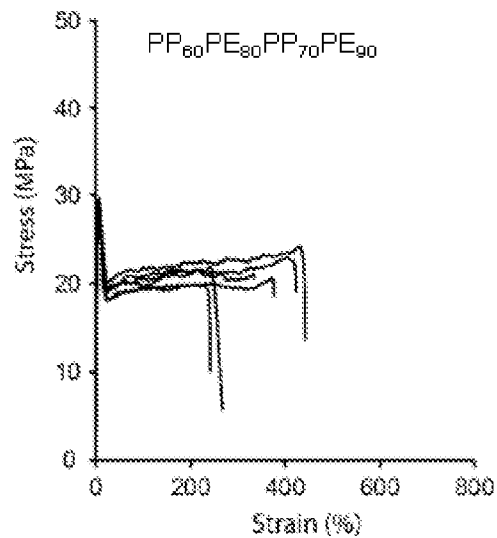
FIG. 22C
