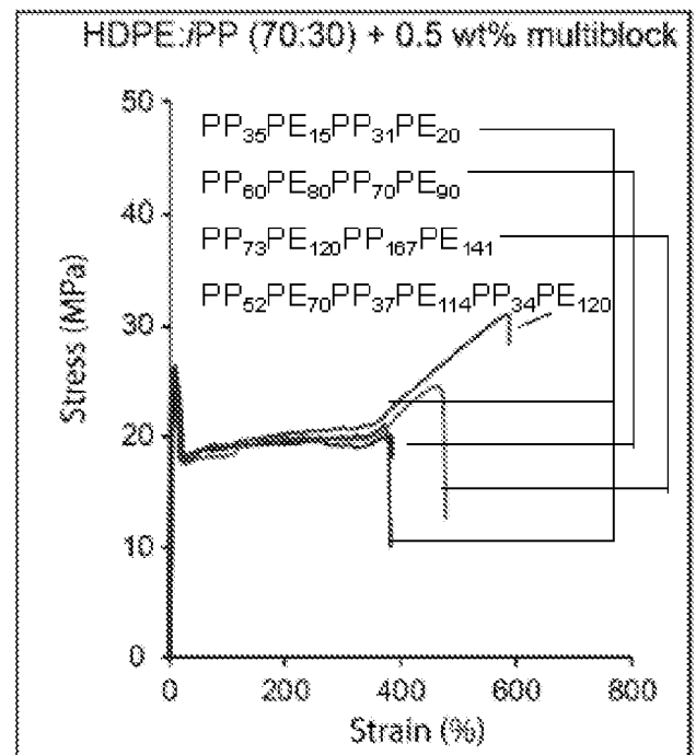
FIG. 20B
