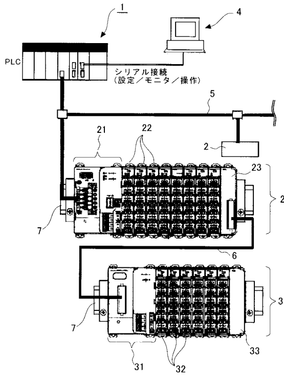
本発明が適用されるPLCシステム全体の構成図
