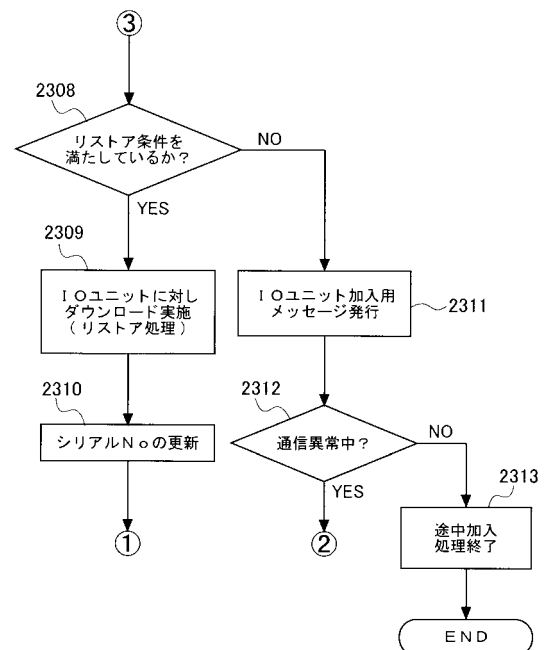
通信ユニットの途中加入処理を示すフローチャート（その２）
