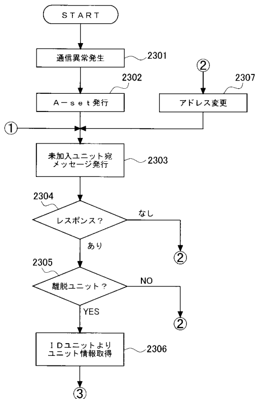
通信ユニットの途中加入処理を示すフローチャート（その１）
