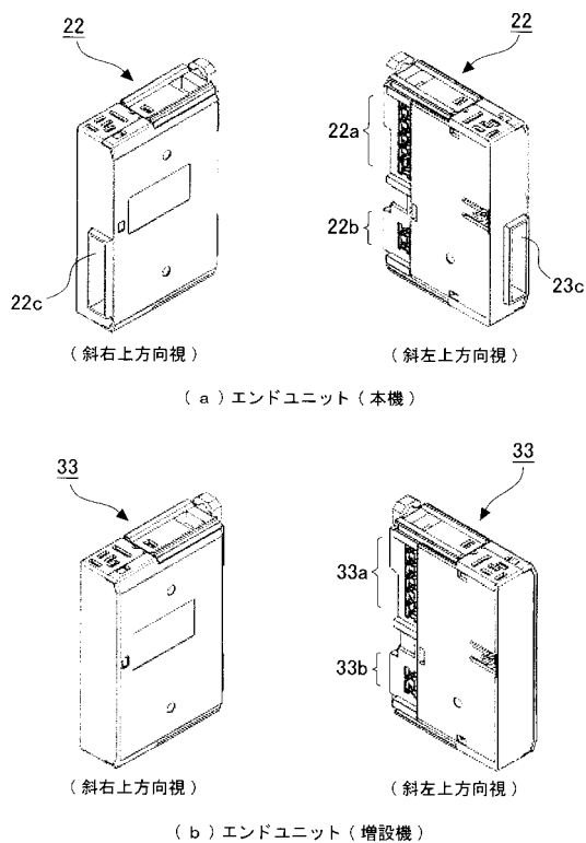
エンドユニットの外観を示す斜視図
