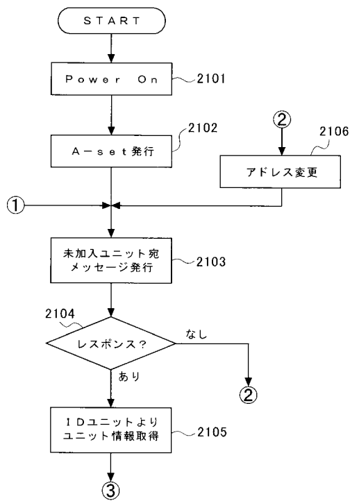
通信ユニットの初期加入処理を示すフローチャート（その１）
