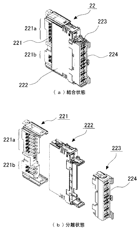
I/Oユニットの斜視図（斜左上方向視）
