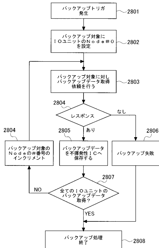
通信ユニットのバックアップ処理を示すフローチャート
