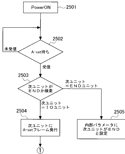
1 / Oユニットの初期加入処理を示すフローチャート（その1）
