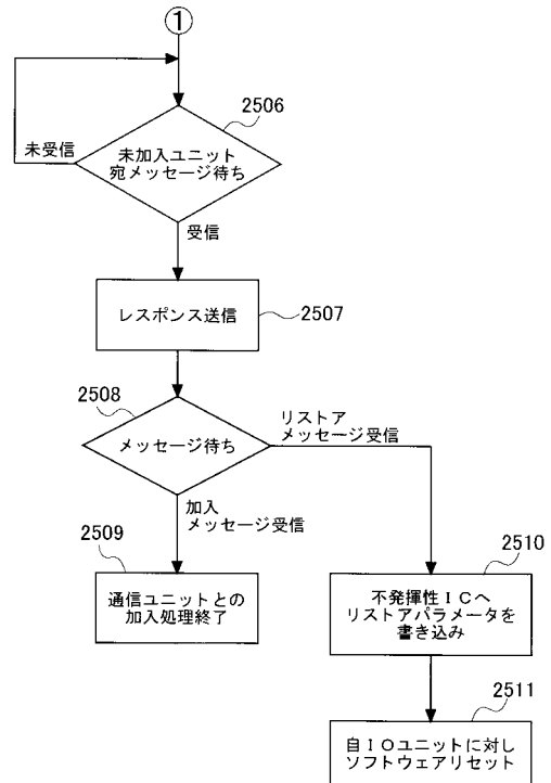
1 / Oユニットの初期加入処理を示すフローチャート（その2）
