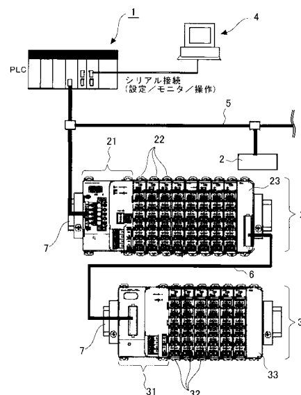
本発明が適用されるPLCシステム全体の構成図
