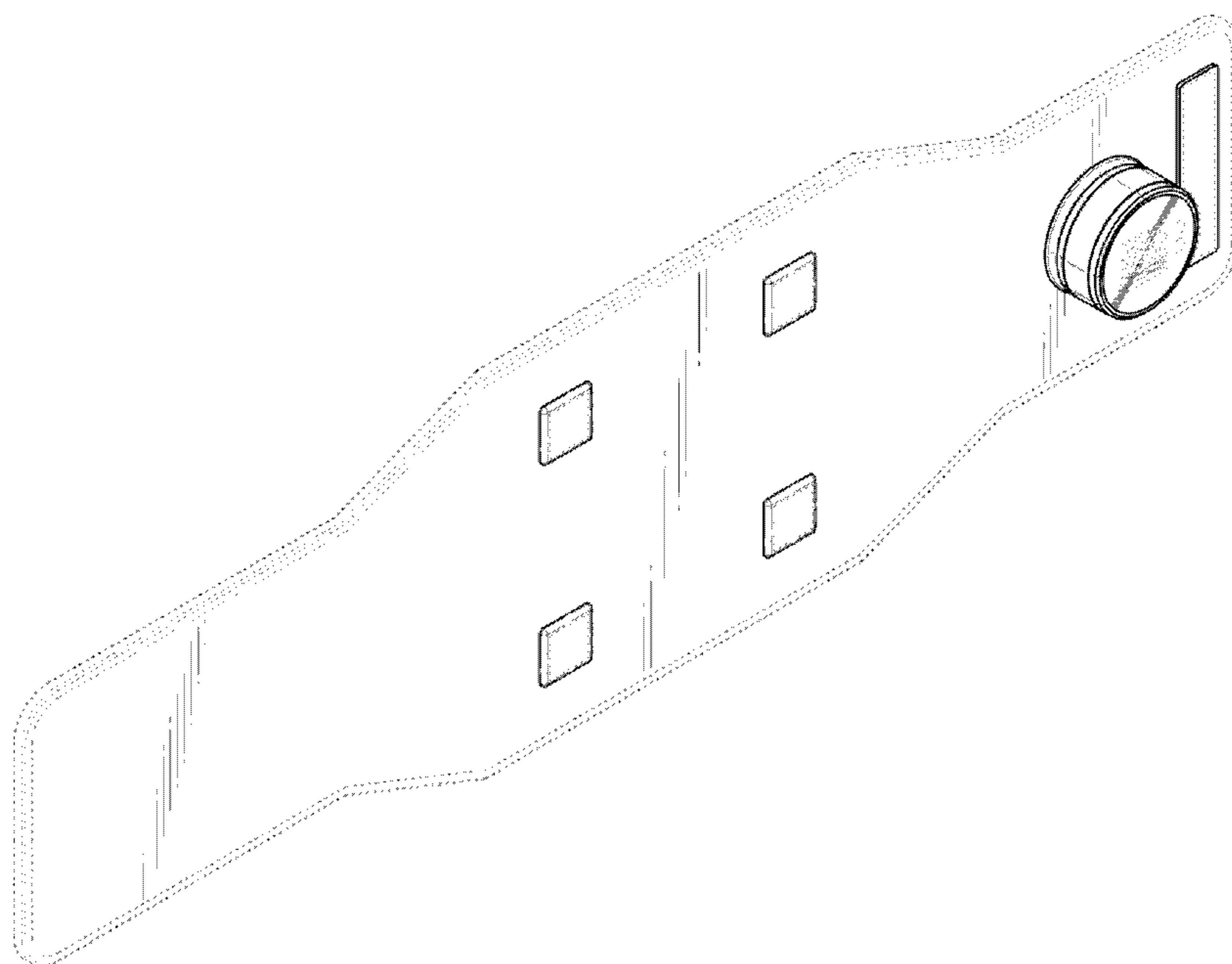
【立體圖1】
