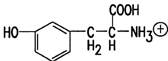
TYROSINE
