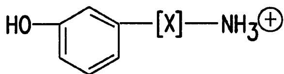
NTox
