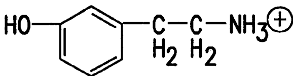
TYRAMINE
