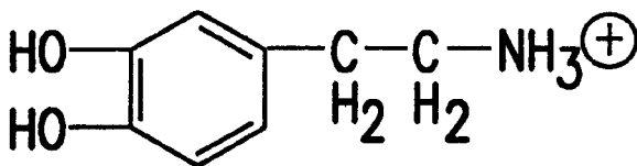
DOPAMINE
