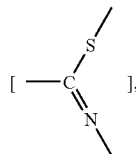
1,3,4-triazol-2,5-ylens
