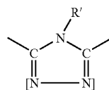
1,3,4-triazol-2,5-ylens
