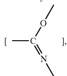
nitrilomethyleneiminos
