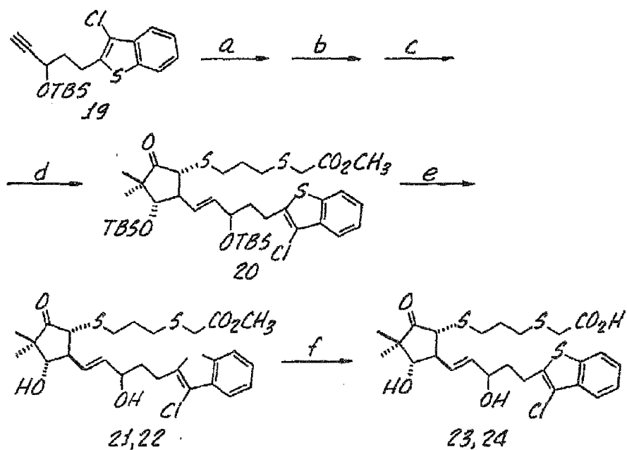
Fig. 5. (SCHEME 5)
