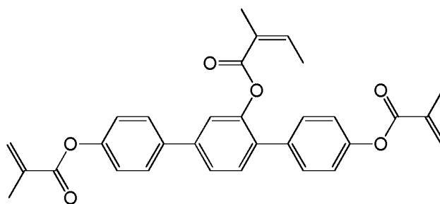
(1-3-23)
