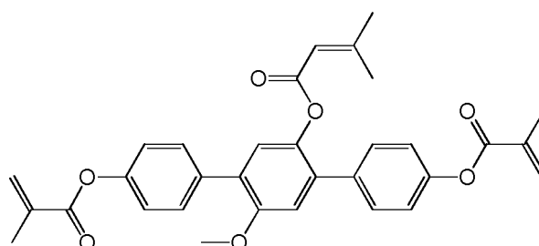
(1-3-30)
