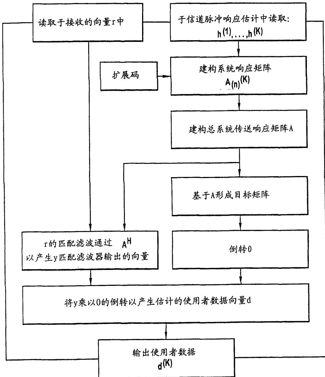
图 5 (现有技术)
