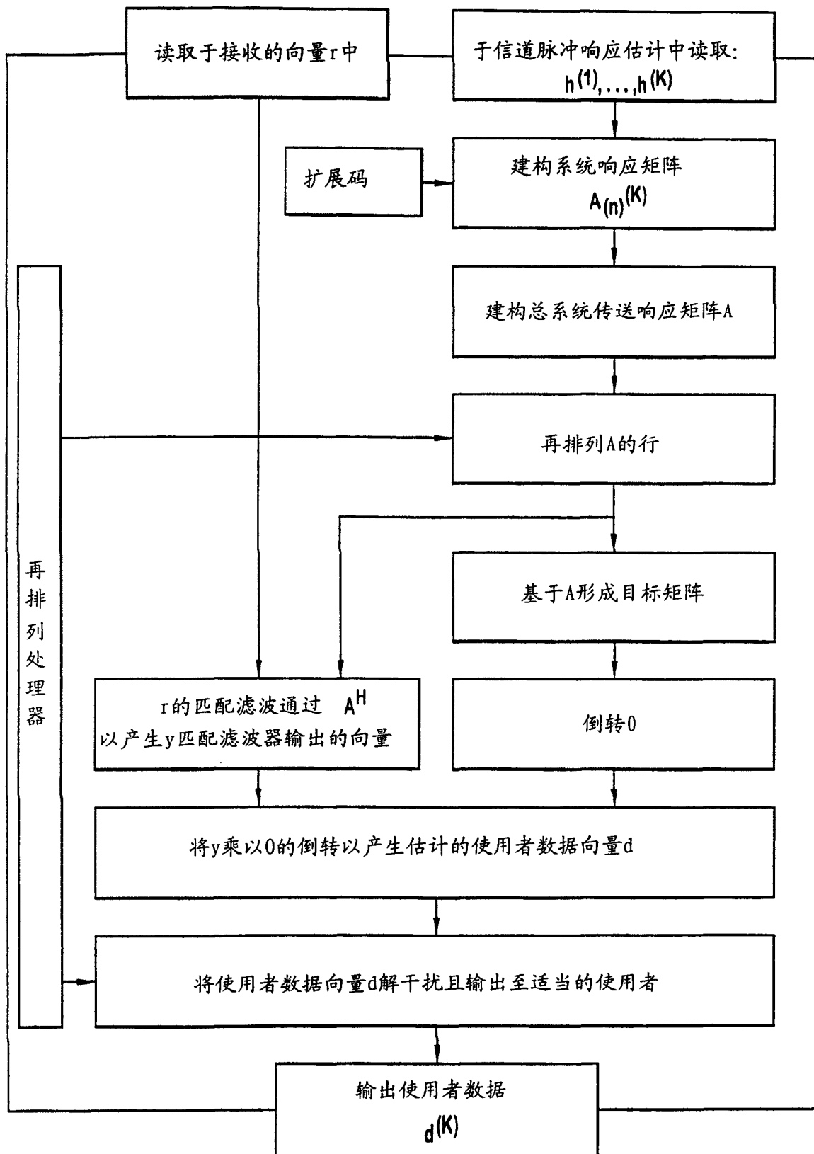
图 6 (现有技术)
