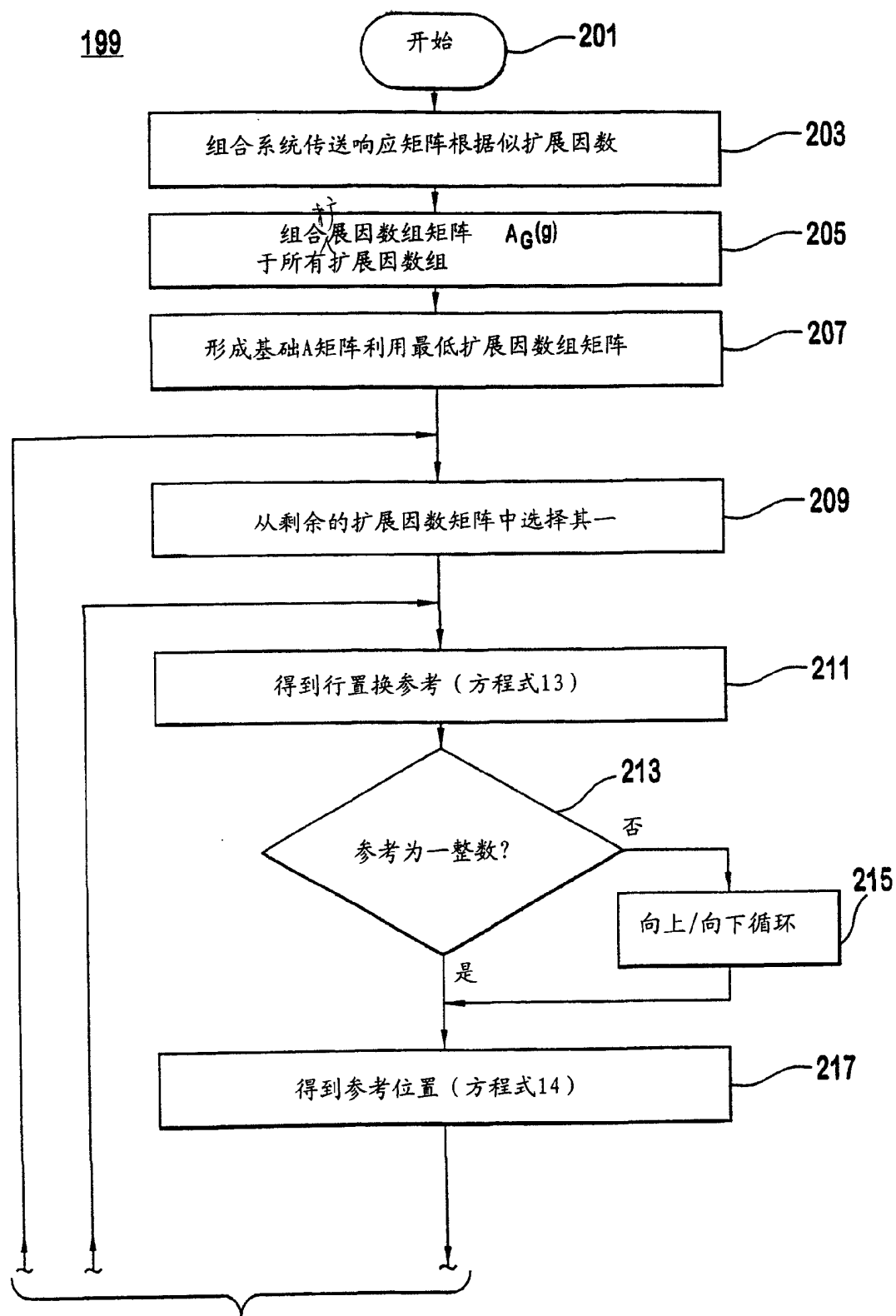
图10B
