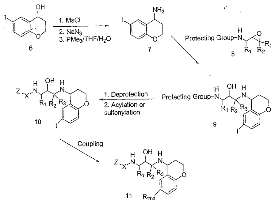
Scheme VI
