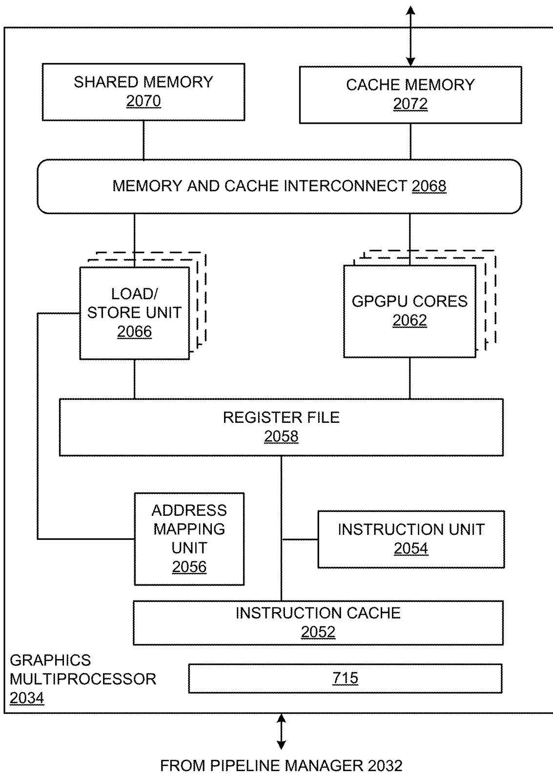
FIG. 20D
