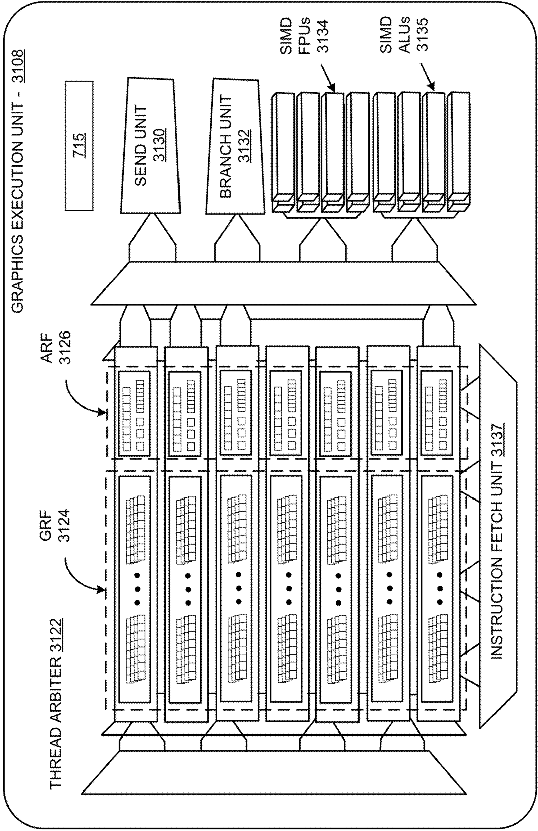
FIG. 31B
