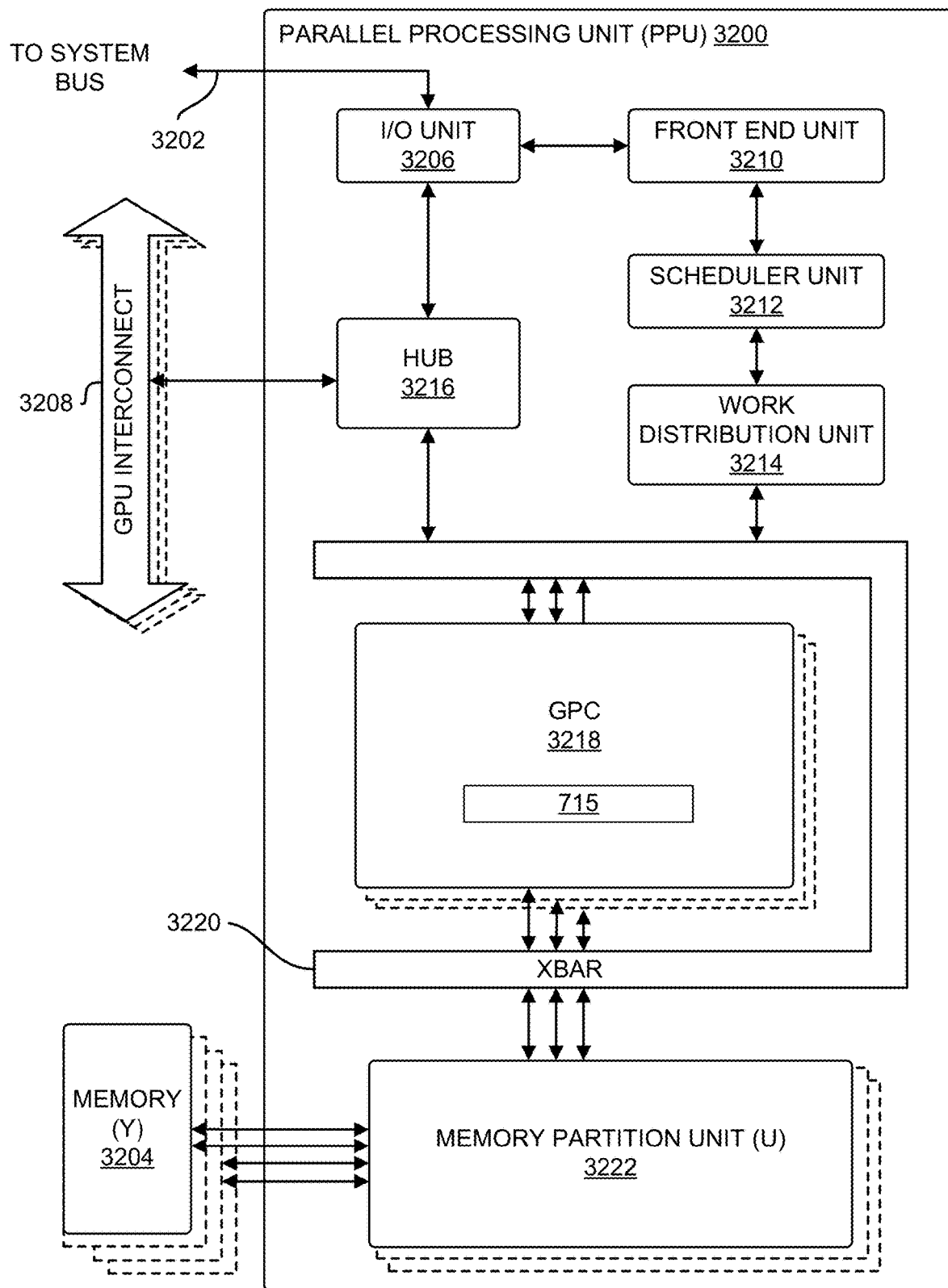
FIG. 32
