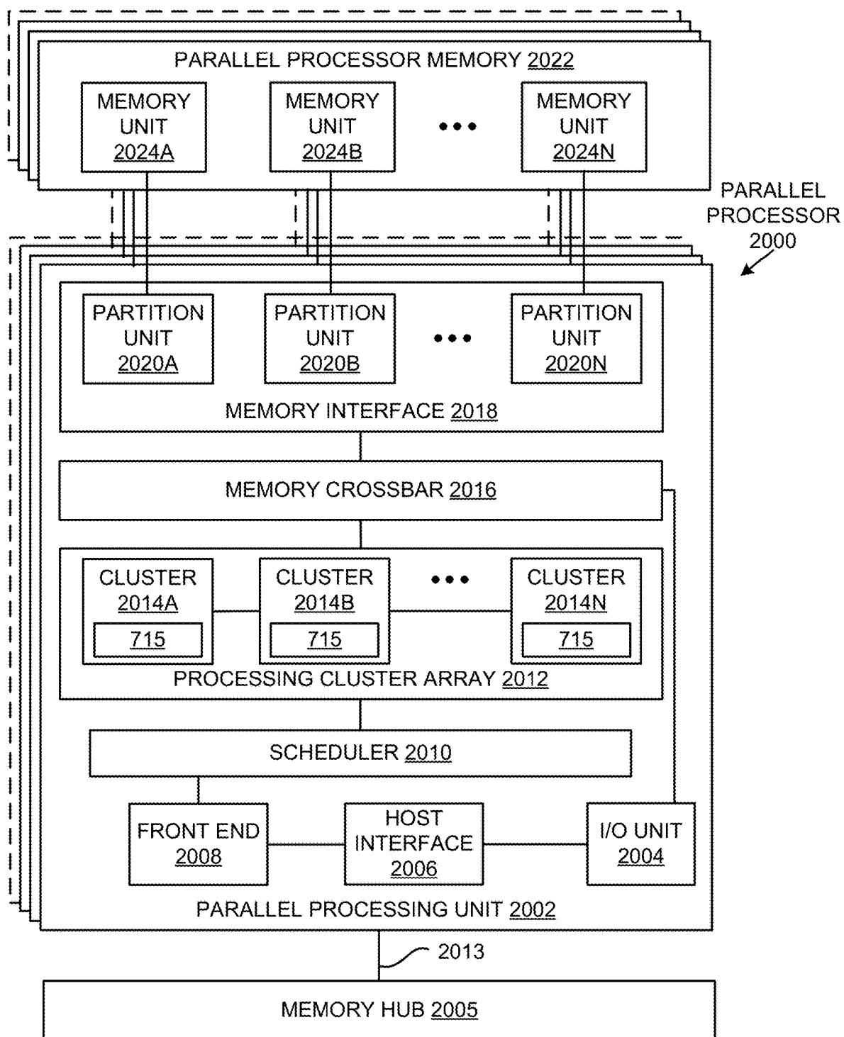
FIG. 20A
