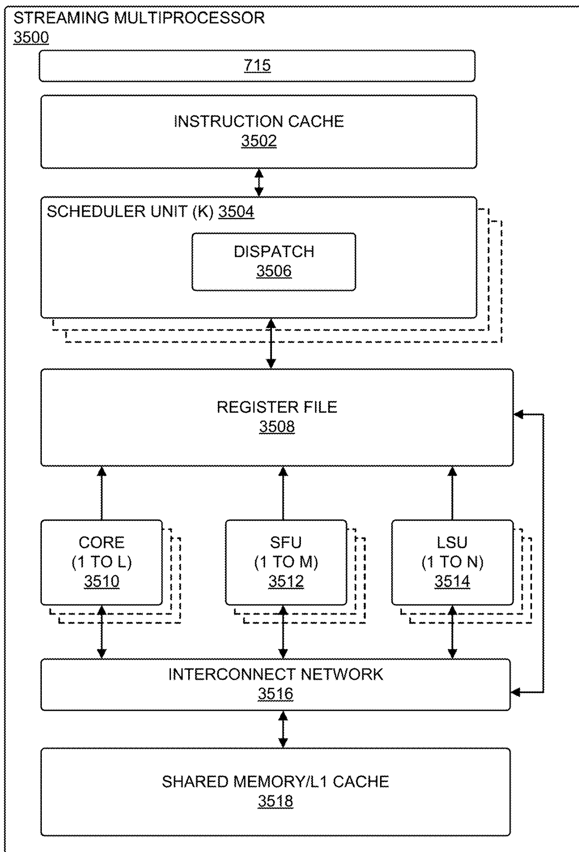
FIG. 35
