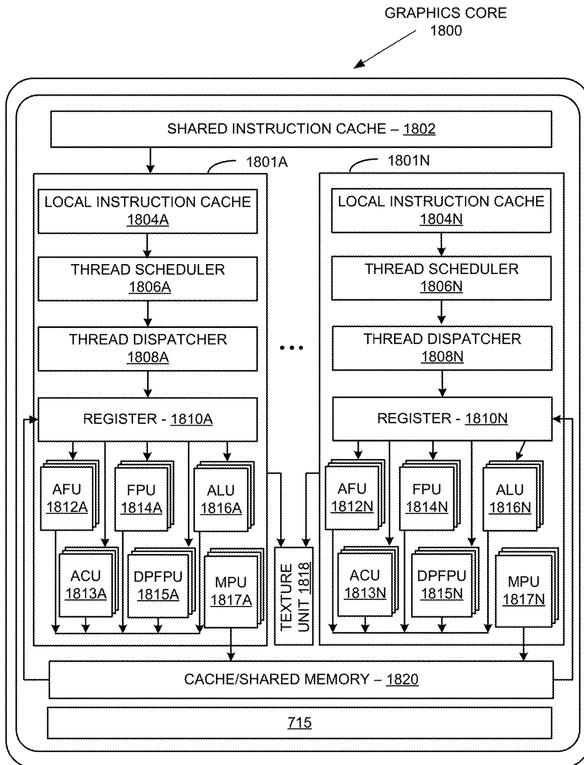
FIG. 18A
