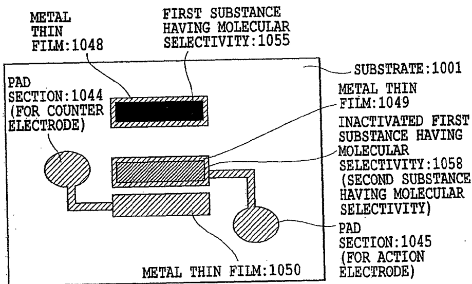
FIG.20A
