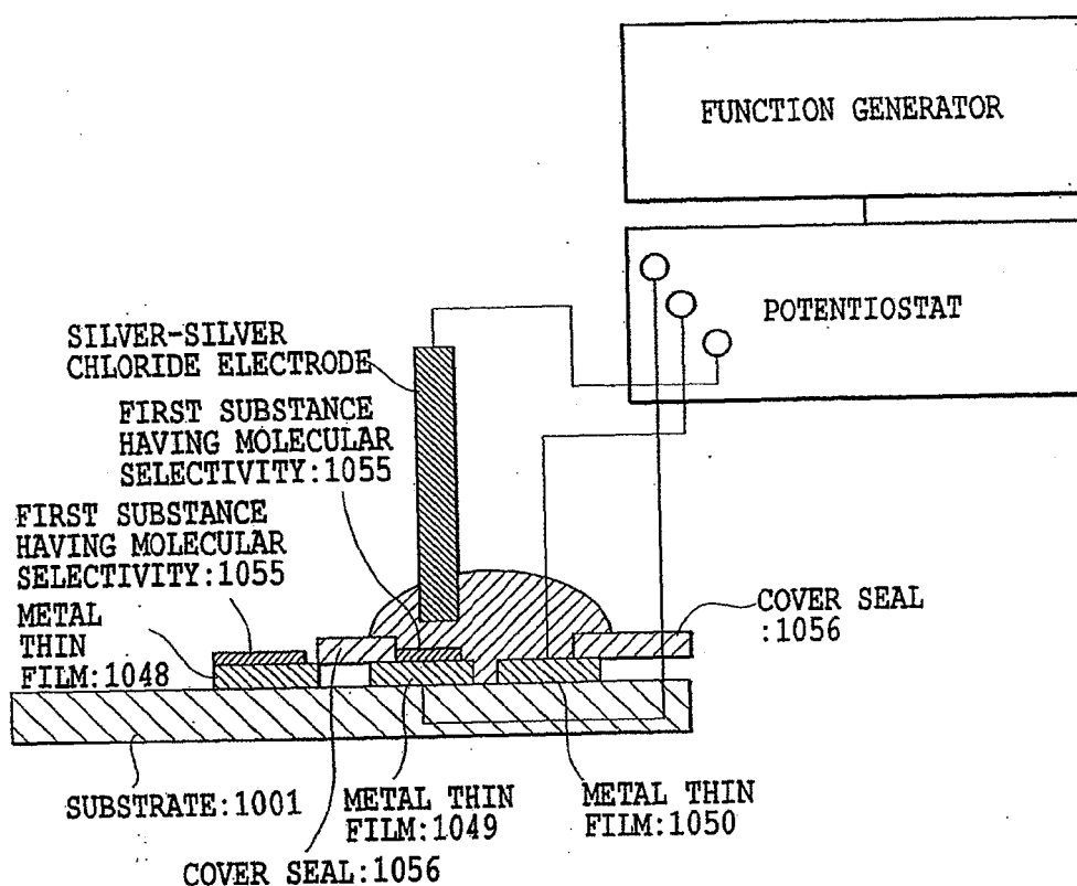
FIG.20A
