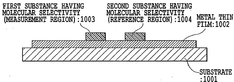
FIG.16B
