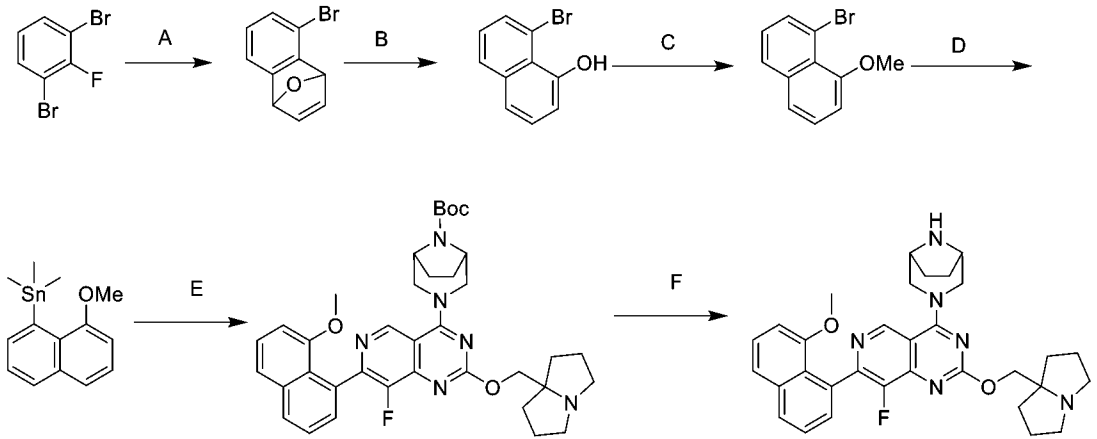
4-((1R,5S)-3,8-二氮雜雙環[3.2.1]辛-3-基)-8-氟-2-((六氫-1H-吡喃-7a-基)甲氧基)-7-(8-甲氧基萆-1-基)吡啶并[4,3-d]嘧啶
