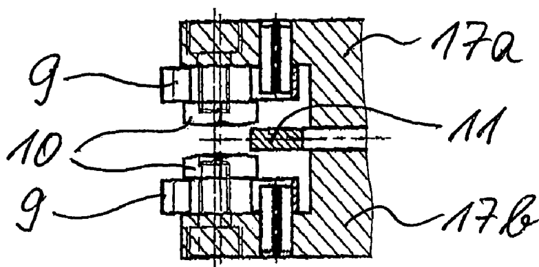
Schnitt D-D Section Cut D-D
