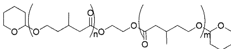
結構式 (III)
