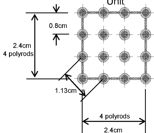
16 Element Array
