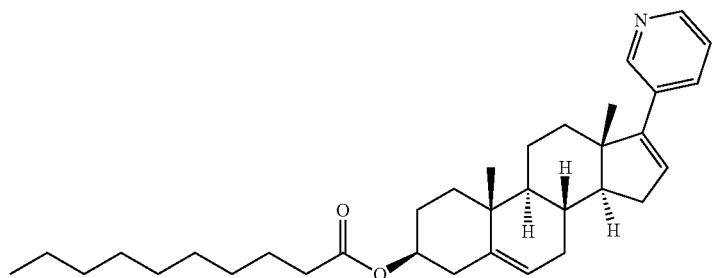
abiraterone decanoate
