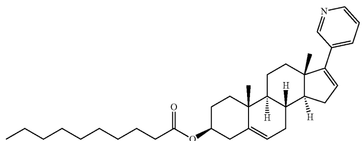
abiraterone decanoate
