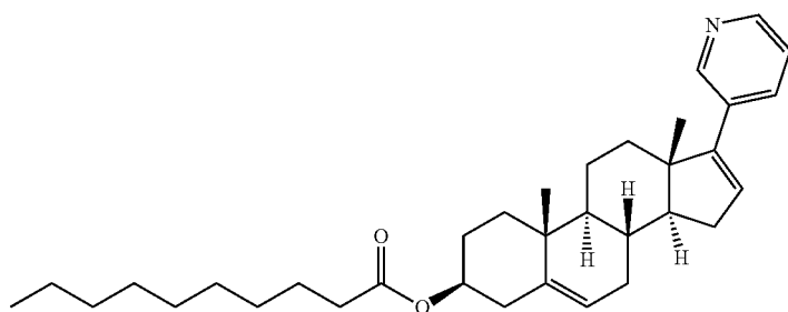
abiraterone decanoate
