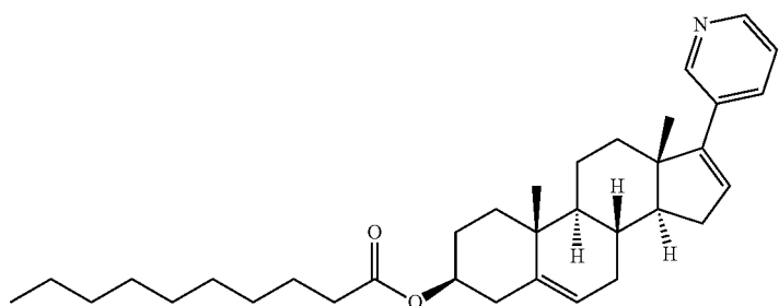
abiraterone decanoate
