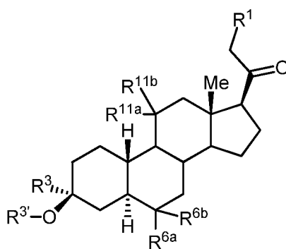
(III-b2)
