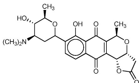
medermycin (V),
