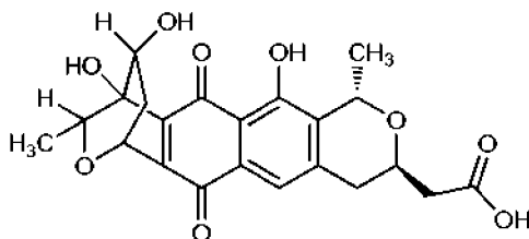
Dérivé 2 (VIII),
