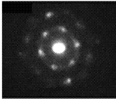
CAAC-OS
