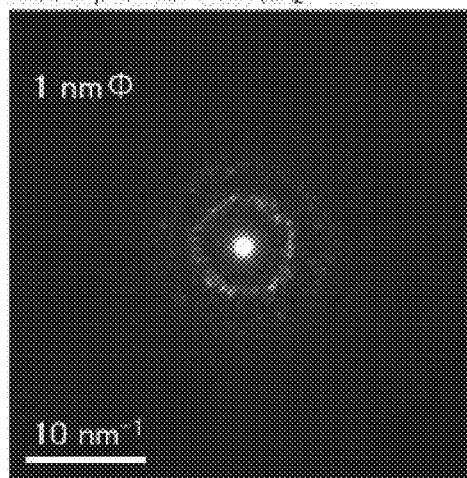
FIG. 25B Sample X3: R.T., O 2 ≅10%
