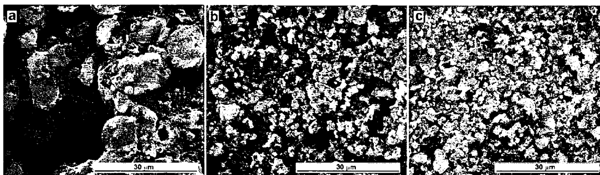
Fig. 2. Zdjęcia wykonane za pomocą skaningowego mikroskopu elektronowego (SEM) dla następujących próbek: (a) CNOs, (b) CNOs/4-aminobenzylamina, (c) CNOs/pochodna.
