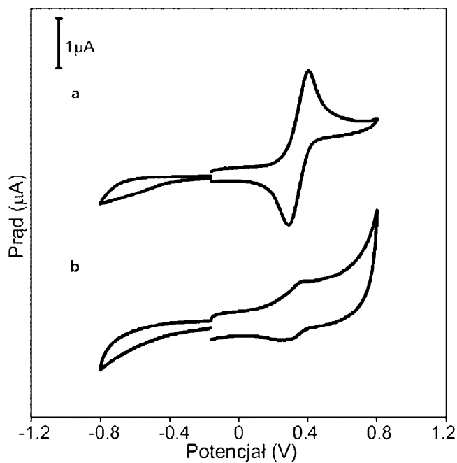
Fig. 6. Krzywe chronowoltamperometryczne zarejestrowane w układzie trójelektrodowym w mieszaninie acetonitryl/toluen (1:4, v/v) w zakresie potencjałów -1,0 ÷ 1,0 V przy stałej szybkości polaryzacji 50 mV/s dla następujących próbek: (a) ferrocenowy kwas karboksylowy – Fc-COOH, (b) CNOs/amid/Fc.
