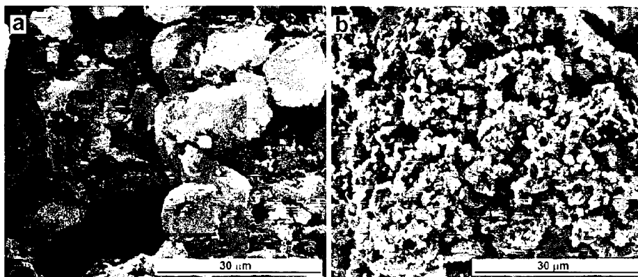
Fig. 7. Zdjęcie 0,5 mg/ml roztworu wielościennych fulerenów w toluenie: (a) CNOs, (b) CNOs/maleimid.
