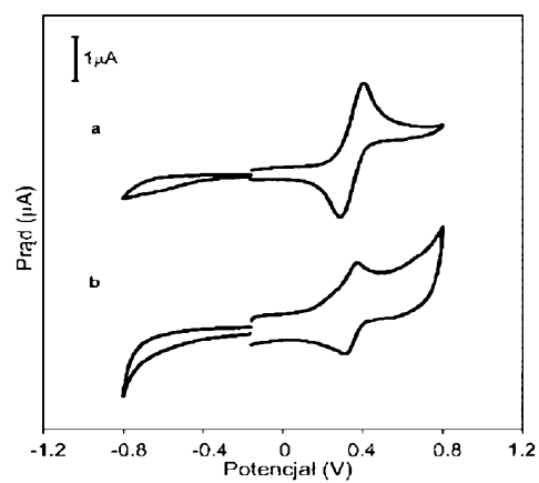
Fig. 9. Krzywe chronowoltamperometryczne zarejestrowane w układzie trójelektrodowym w mieszaninie acetonitryl/toluen (1:4, v/v) w zakresie potencjałów -1,0 ÷ 1,0 V przy stałej szybkości polaryzacji 50 mV/s dla następujących próbek: (a) ferrocenowy kwas karboksylowy – Fc-COOH, (b) CNOs/maleimid/Fc.
