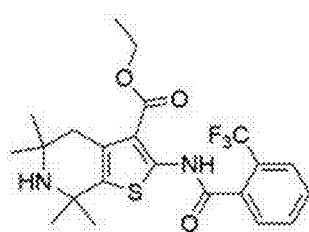
GP1-02; MW = 455
