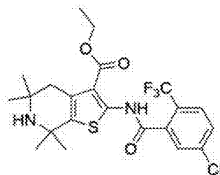
GP1-03; MW = 488
