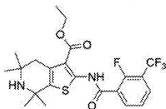
GP1-04; MW = 472
