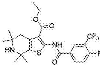
GP1-05; MW = 472
