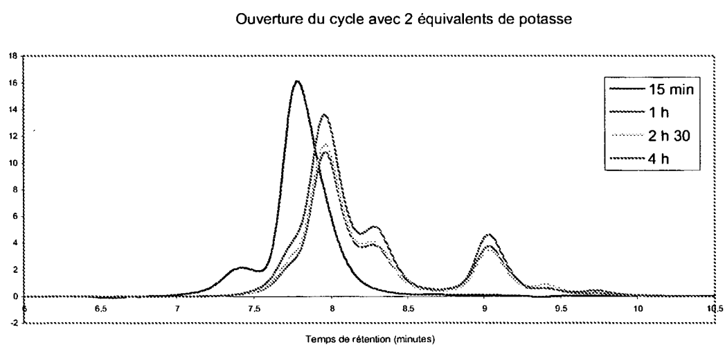
Figure 3 : Chromatogrammes avec 2 équivalents de potasse par rapport au cycle
