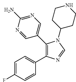
SB 220025
