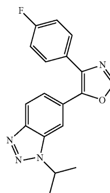
4-(4-fluorophenyl)-5-(1-isopropyl-1H-benzo[d][1,2,3]triazol-6-yl)oxazole
