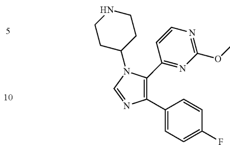
SB-242235
