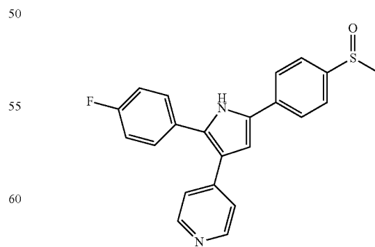
L-167307
