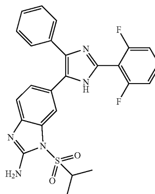
6-(2-(2,6-difluorophenyl)-4-phenyl-1H-imidazol-5-yl)-1-(isopropylsulfonyl)-1H-benzo[d]imidazol-2-amine
