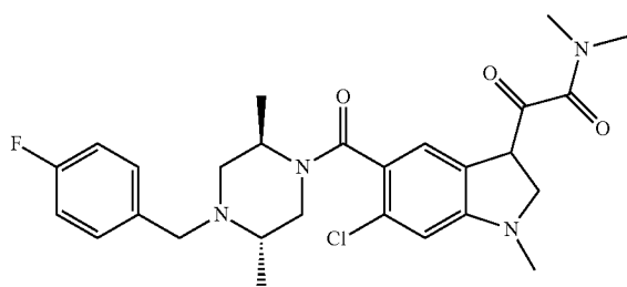
SCIO 469
