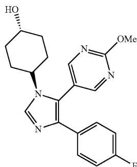
SB 239063
