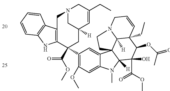
Vinorelbine
