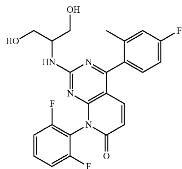
SB-681323
