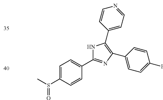
SB-203580
