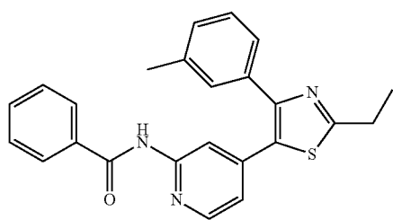
TAK-715
