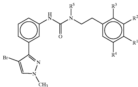
N-[3-(4-bromo-1-methylpyrazol-3-yl)phenyl][2-(4-methoxyphenyl)ethyl]amino] carboxamide
