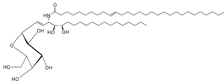
trans-(A-1),
