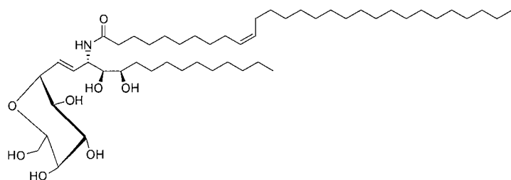
cis-(A-1)
