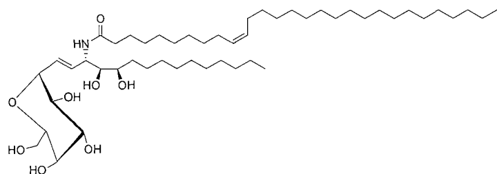
cis-(A-1),
