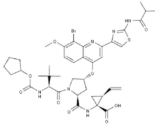
BI-201335
