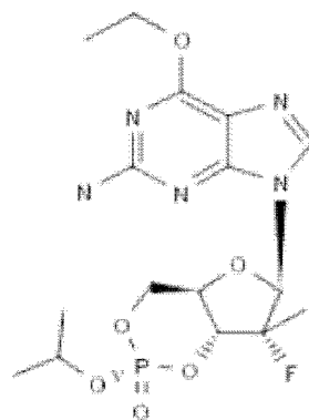
PSI-352938
