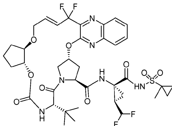
化合物1
