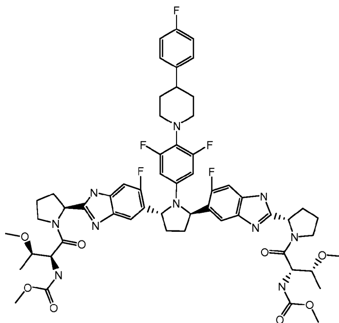
化合物2
