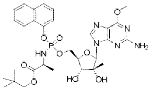
INX-189
