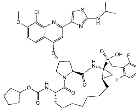
GS-9256
