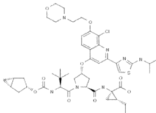
GS-9451
