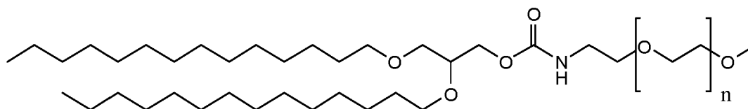
mPEG-2000-DMG
