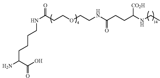
N ε -Lys(PEG4-isoGlu-Palm)
