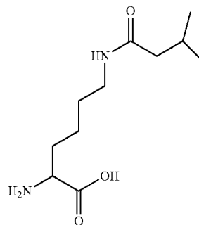
N ε -Lys(IVA)
