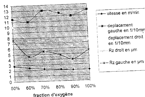
Caractéristique de la coupe (120 A, 10 mm)
