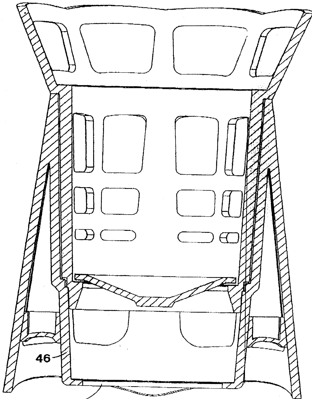
SECTION B-B FIG. 14
