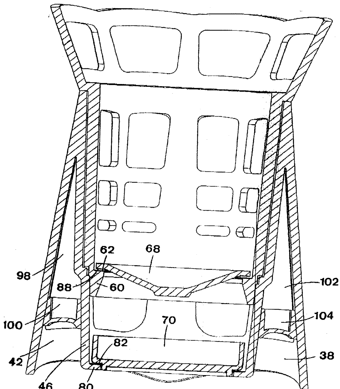
SECTION B-B FIG. 8
