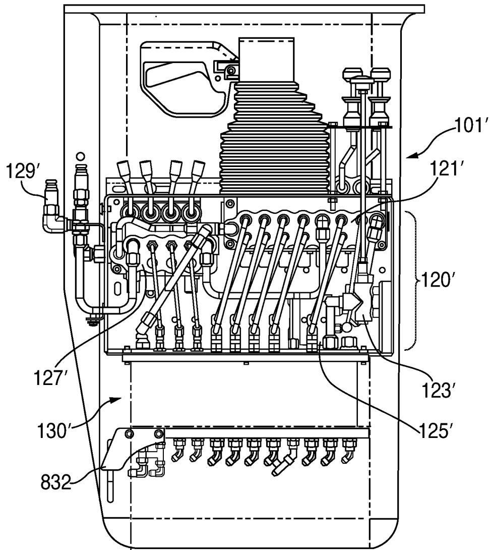
FIG. 8B
