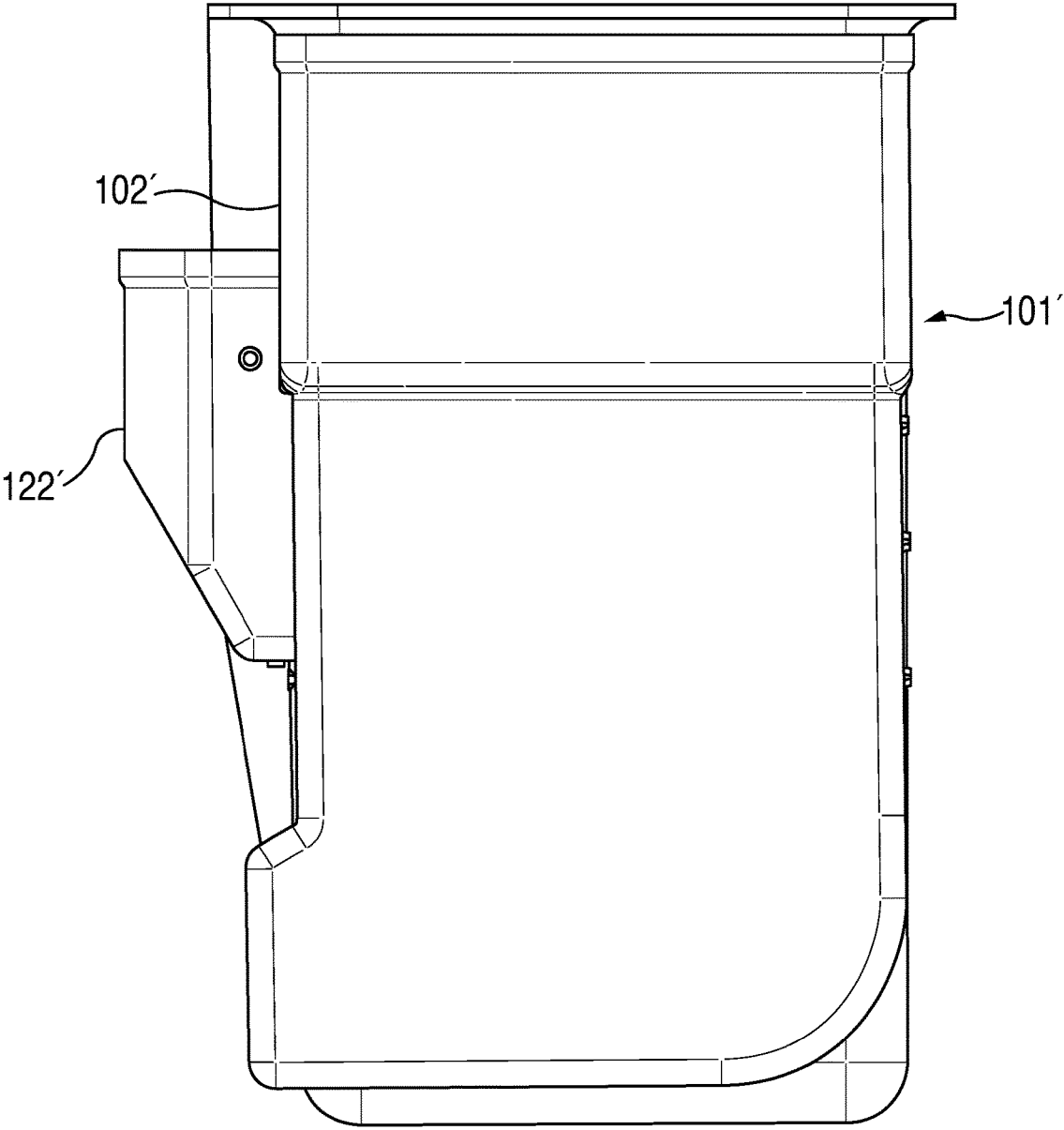
FIG. 8A
