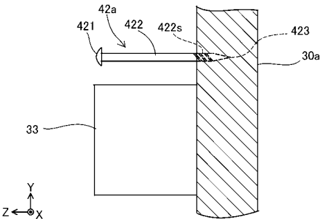
(b) 2-2線矢視断面図
