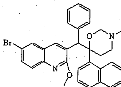
Composto 1
