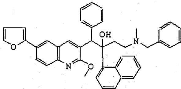
Intermediário 17
