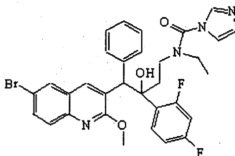
Intermediário 18
