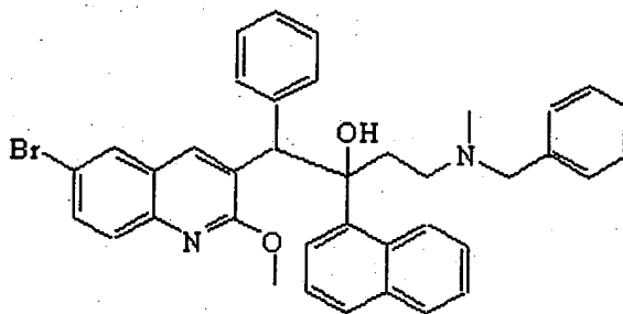
Intermediário 9
