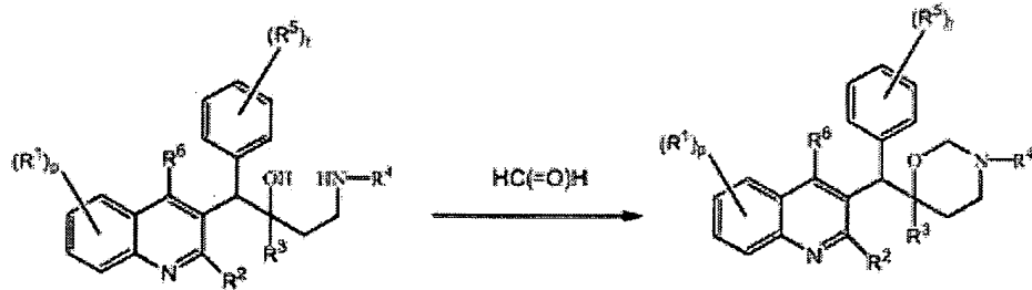
(II-a)
