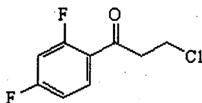
Intermediário 6
