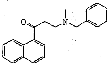
Intermediário 7
