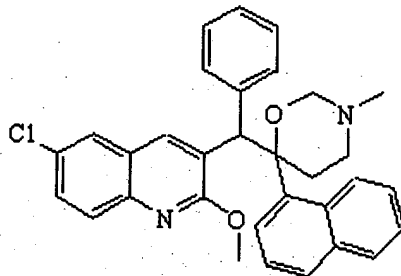
Composto 14
