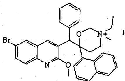
Composto 19
