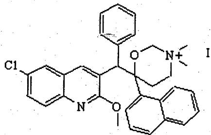
Composto 15
