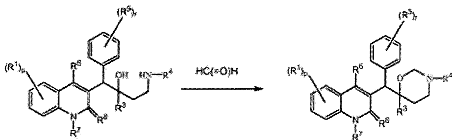
(II-b)
