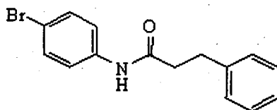
Intermediário 1
