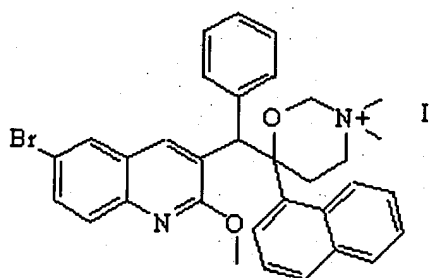
Composto 17
