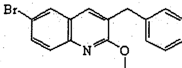
Intermediário 3
