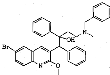
Intermediário 10
