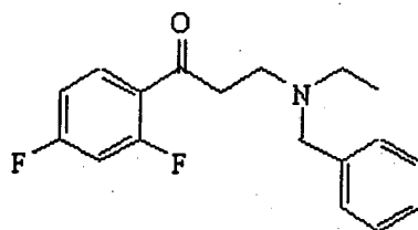
Intermediário 8
