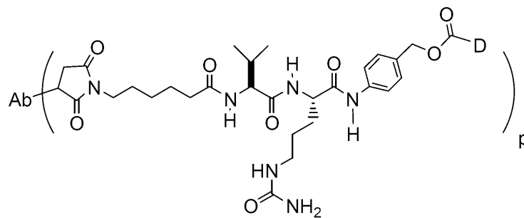
MC-val-cit-PAB
