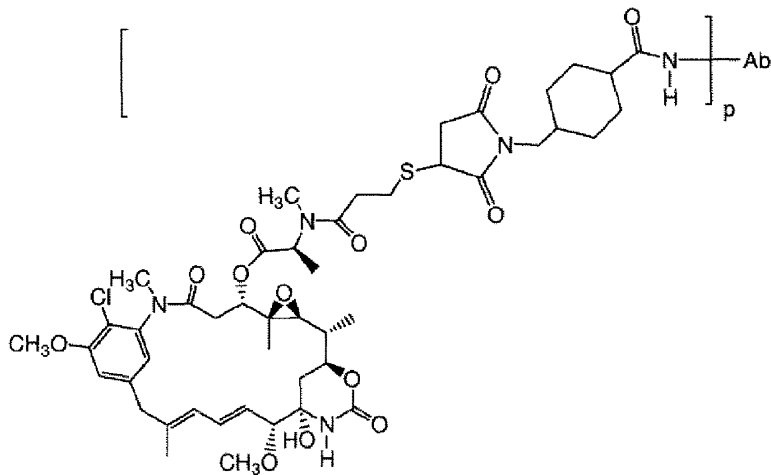
Ab-SPDB-DM4
