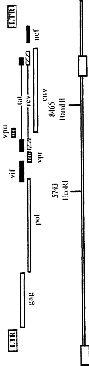
FIG. 11B HIV NL43
