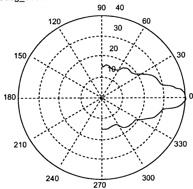
polar_0deg_5000Hz
