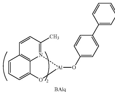
BAlq
