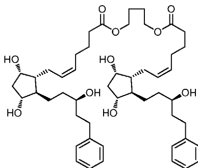
LB-Dimer.
