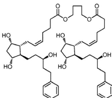
LB-dimère.
