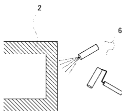
【図2】剥離用皮膜の塗布時の断面図
